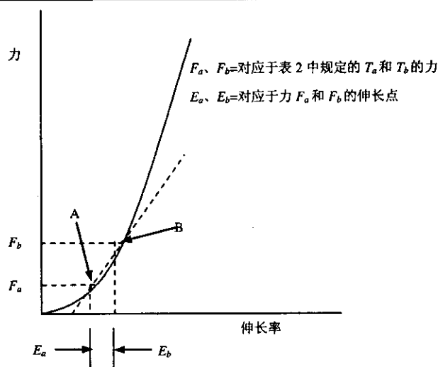
图2 确定拉伸模量的力—伸长率曲线
