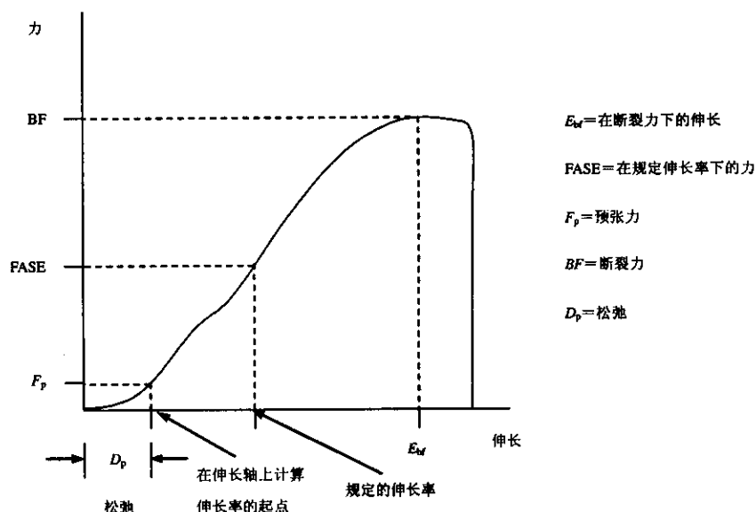
图1 力—伸长曲线
